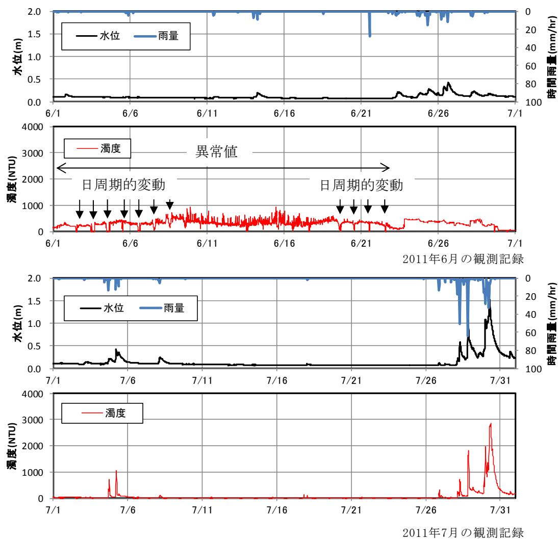
図ー6 観測期間中の特定の時期以降、しばらく継続して一定値を示した後、解消された異常データの例 (上の図は図ー4 の再掲)
