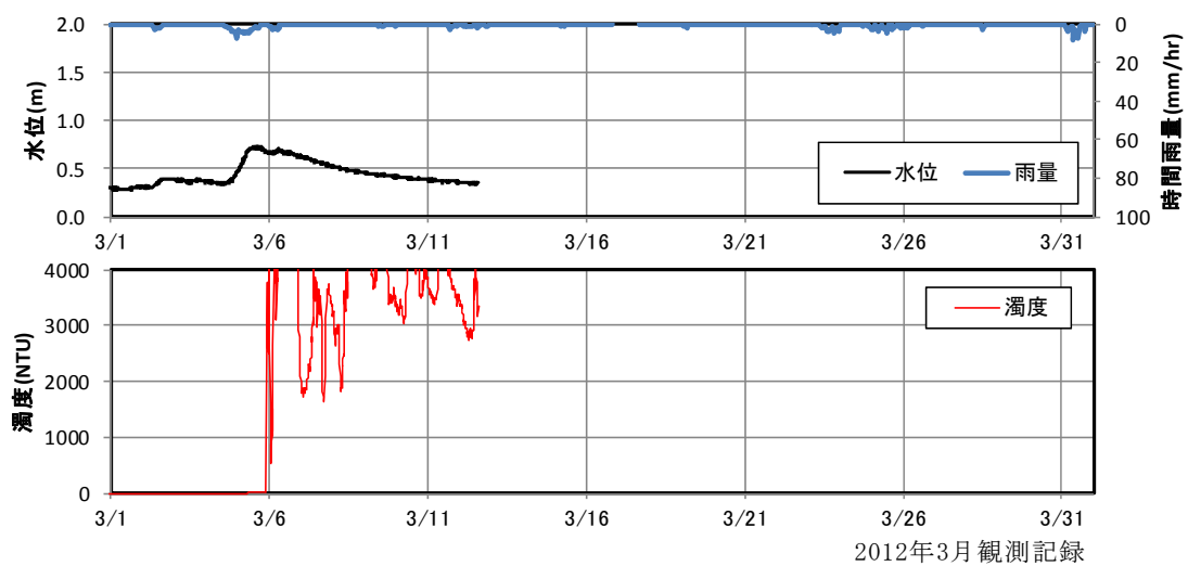
図ー3 観測期間中の特定の時期以降、レンジオーバーを示す異常データの例
