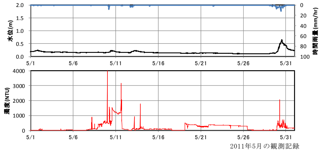
図ー7 洪水時に短期的に水位変動に追従しない異常データの例
