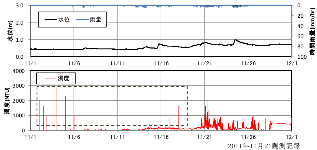
図ー9 ランダムにノイズが入る異常データの例
