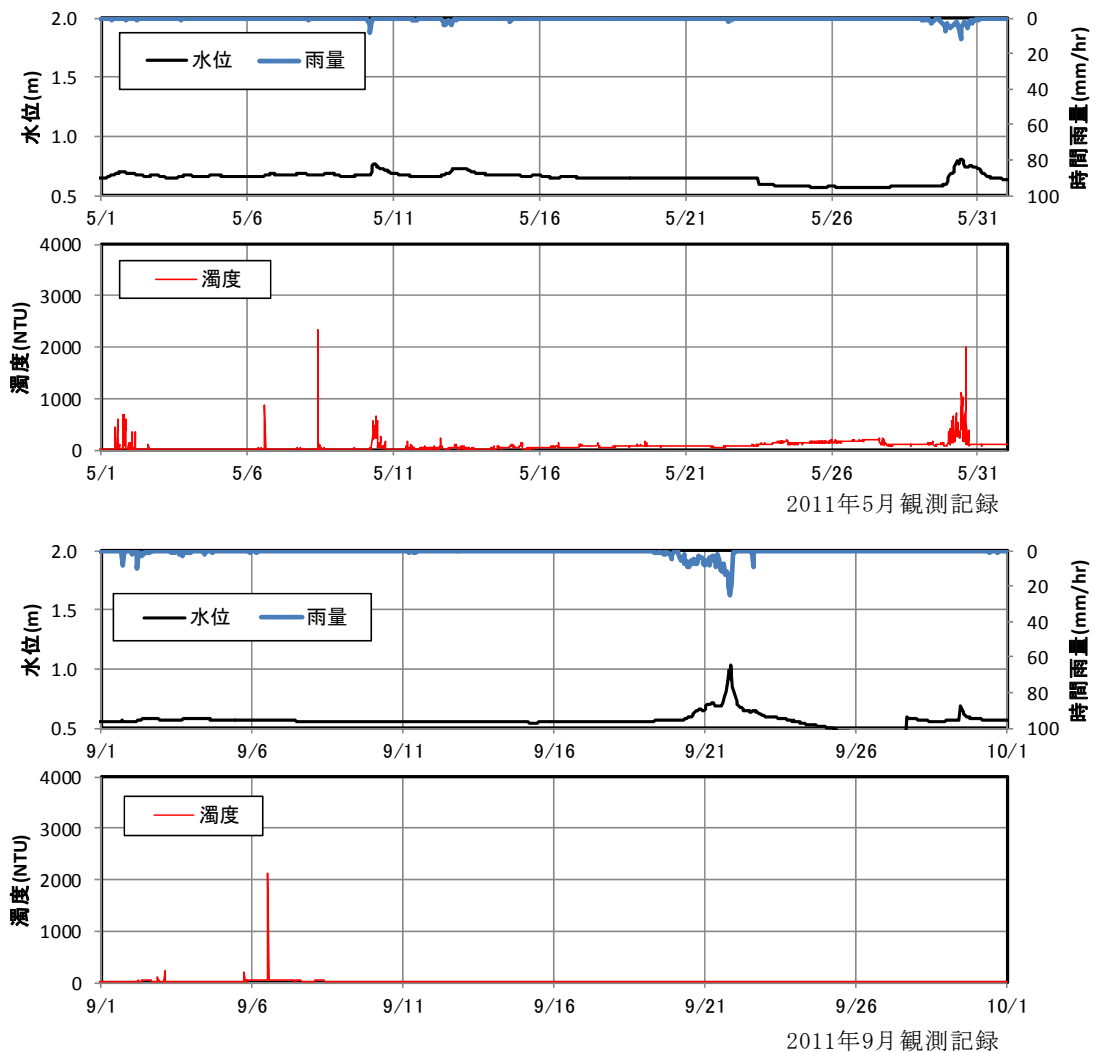
図ー2 観測期間中の特定の時期以降、継続的にゼロに近い値を示す異常データの例
